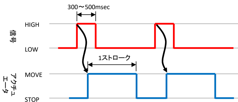
【制御信号チャート】
