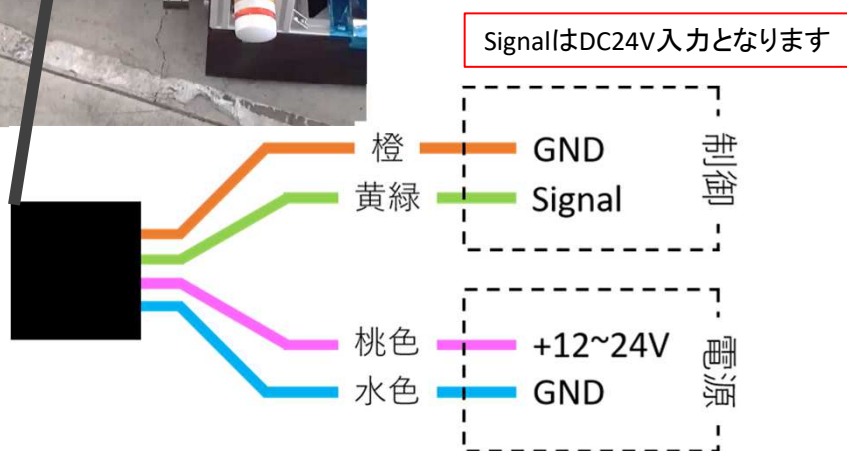
【制御信号チャート】
